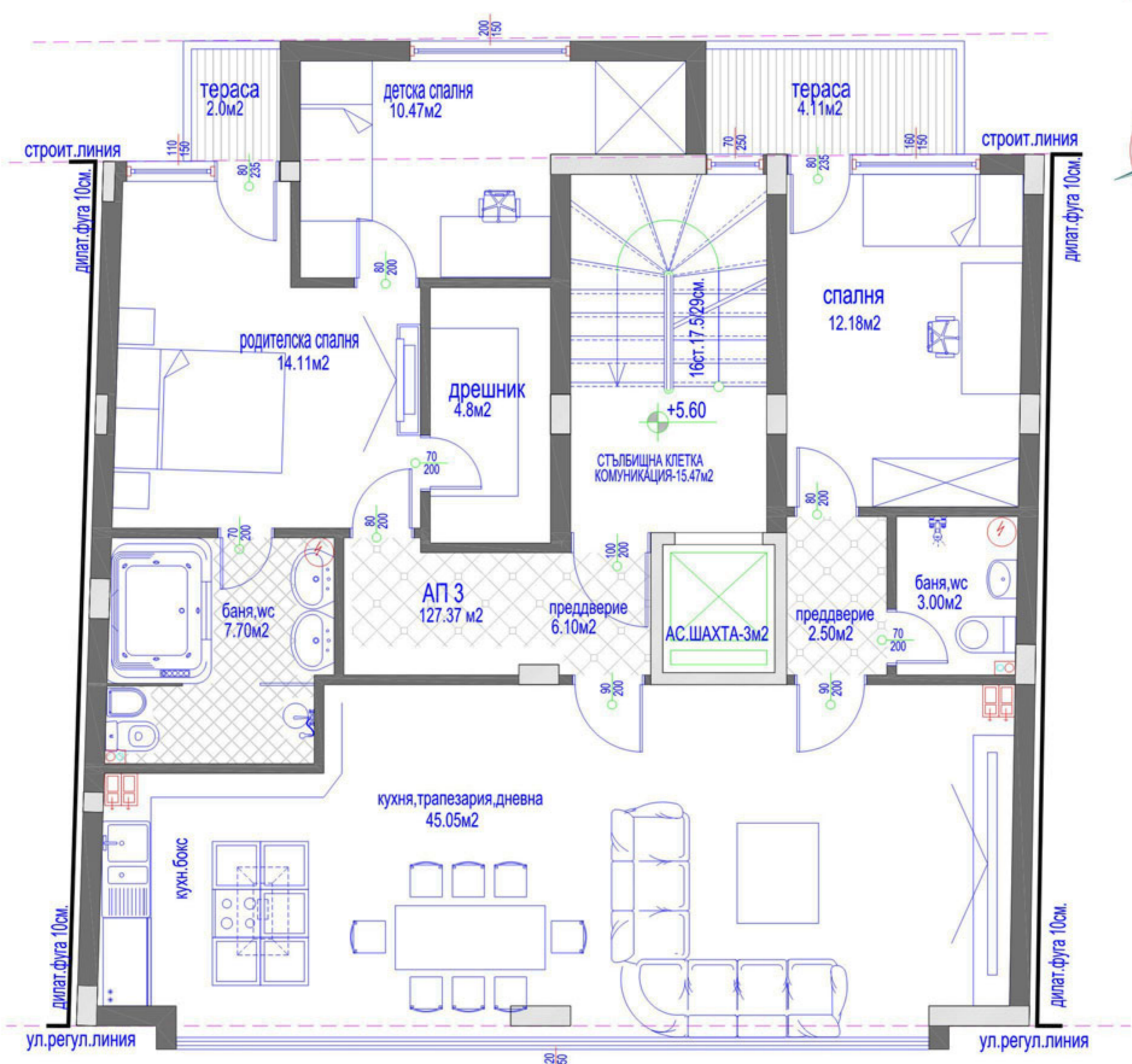
РАЗПРЕДЕЛЕНИЕ ТРЕТИ ЕТАЖ КТ.+5.60 ЗП=146 м2
